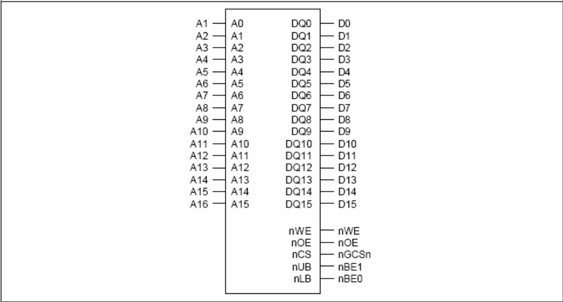
图5-8 16位SRAM存储器接口
