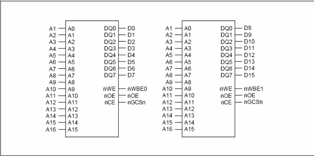
图5-5 2片8位ROM存储器接口
